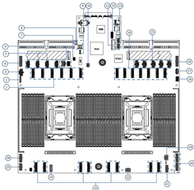
主板图 2-15
