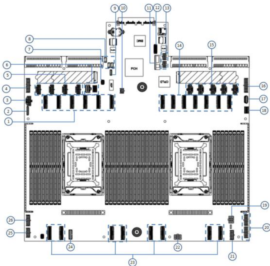
主板图 2-16
