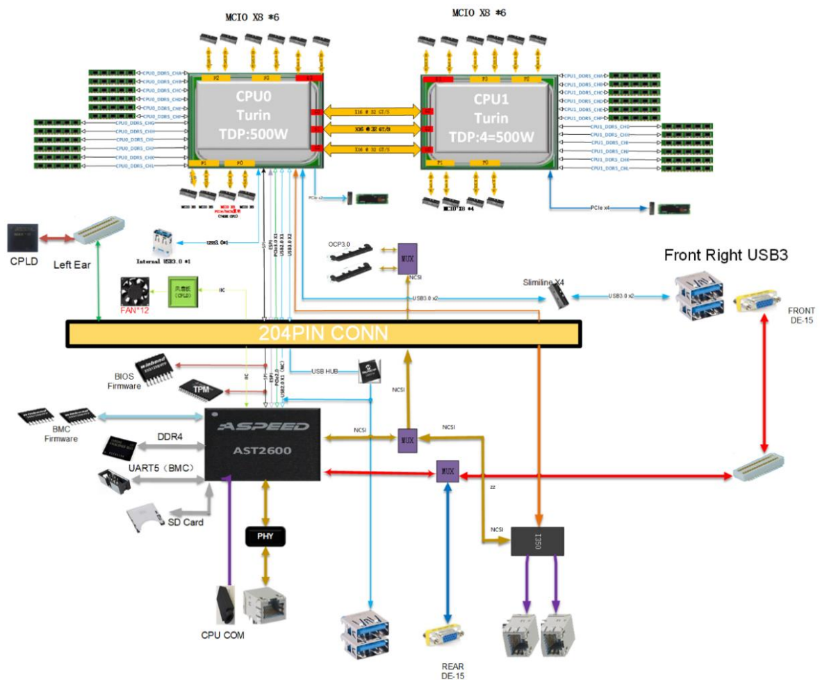
主板逻辑框图
