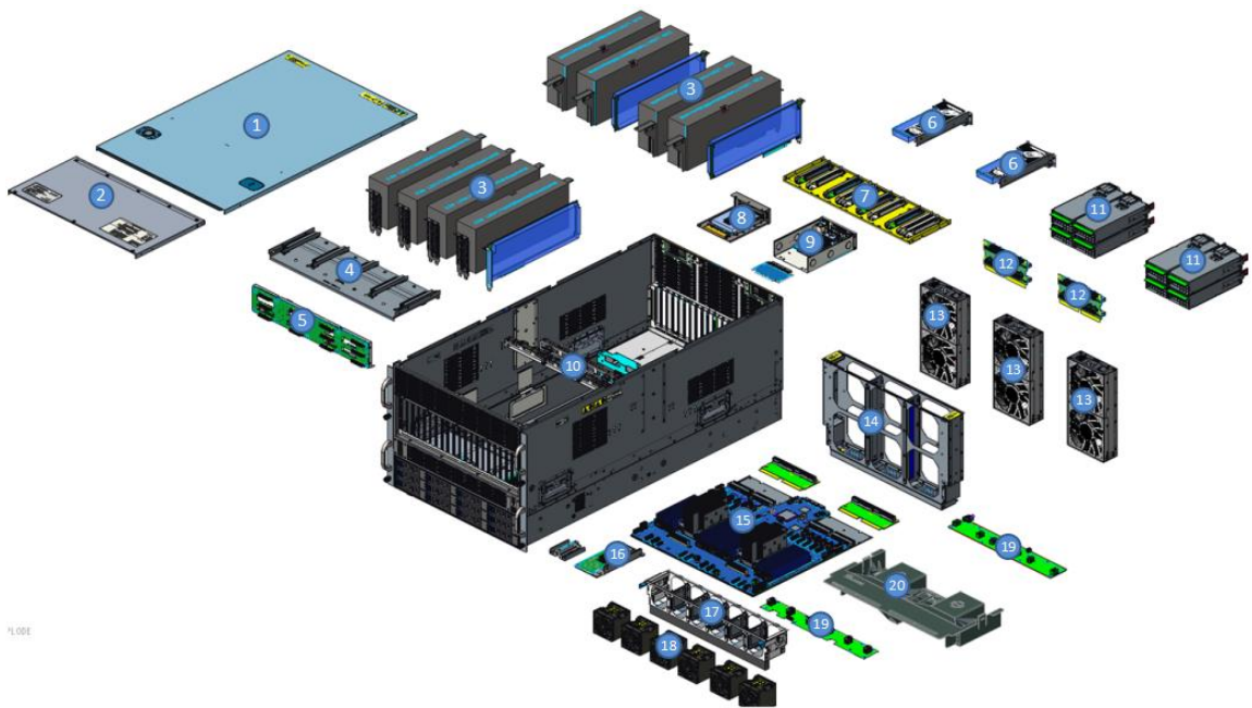
结构爆炸图
