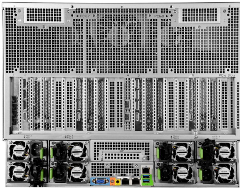
后视图
