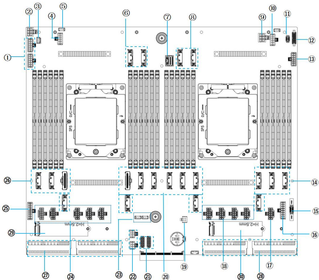
主板图 2-15
