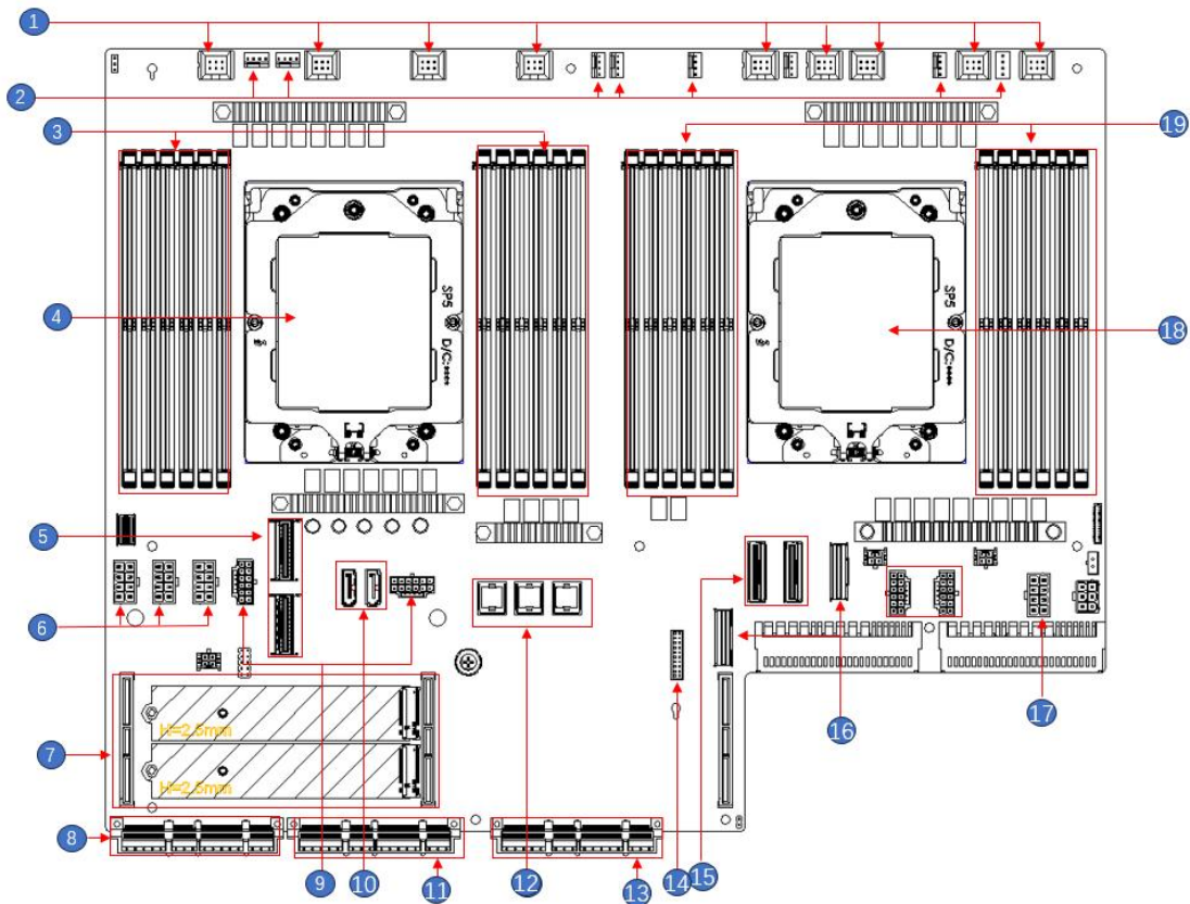
G2DLRO-B 主板图 (2-24)
