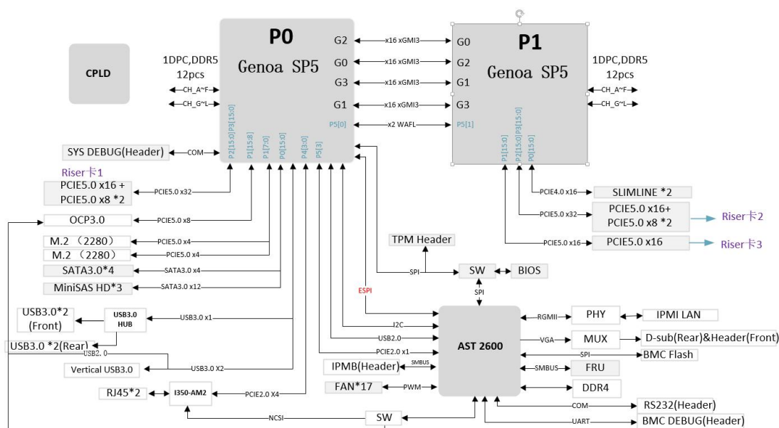
主板逻辑框图 (1-6)
