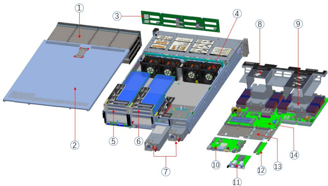
结构图 (1-5)
